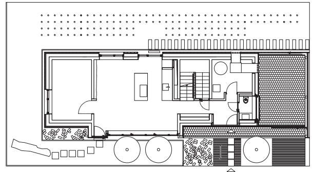
Erdgeschoss
